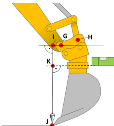
Abb.: 4: Schemabild mit den Messpunkten.
