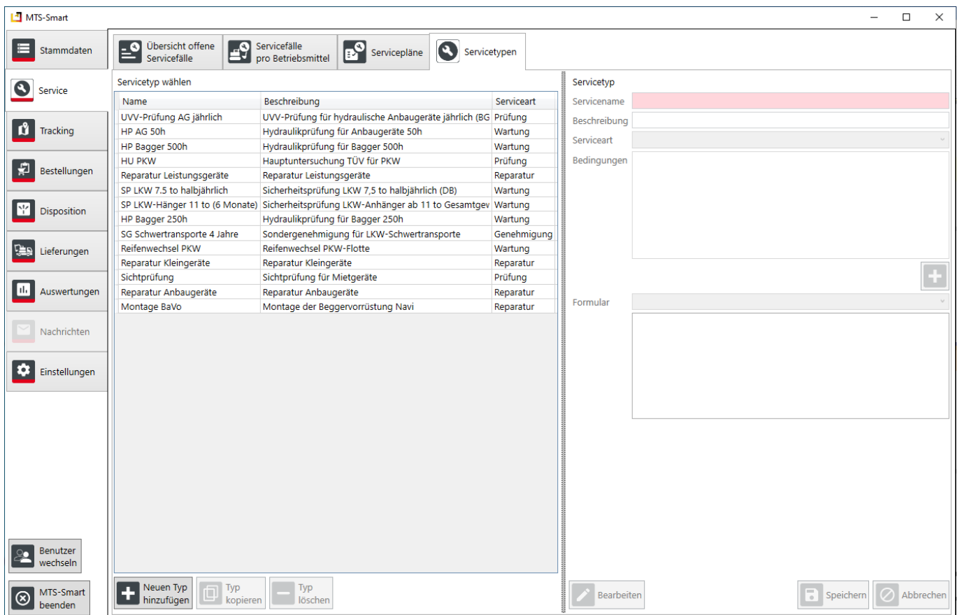
Abbildung 41: Servicetypen
