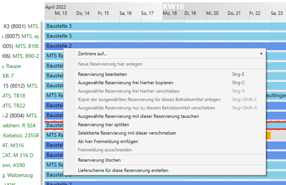
Abbildung 64: Disposition - Kontextmenü
