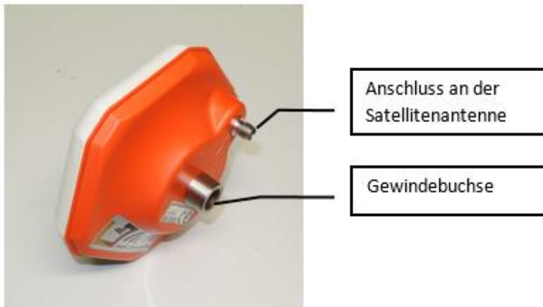
Abb. 12: Satellitenantenne
