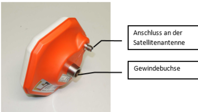
Abb. 12: Satellitenantenne
