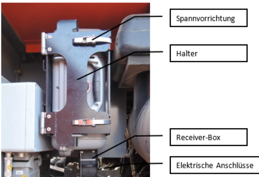
Abb. 5: Receiver-Box in den Halter einbauen (Abbildung ähnlich)
